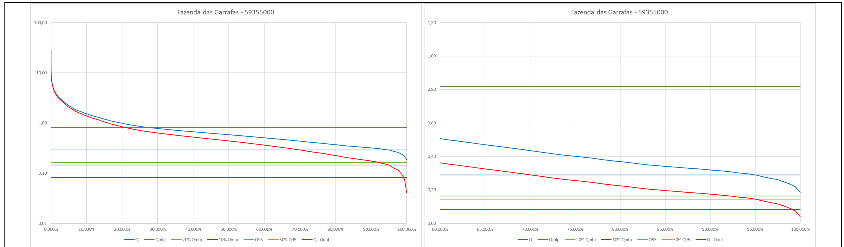
Figura 10.5 - Curva de permanência (vazões naturais e remanescentes) e vazões de Tennant na estação Fazenda das Garrafas (59355000)
